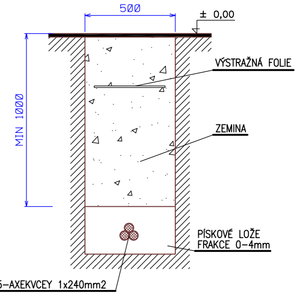
ULOŽENÍ KABELŮ: 1x KVN 35KV
