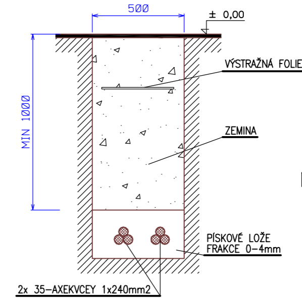
ULOŽENÍ KABELŮ: 2x KVN 35KV
